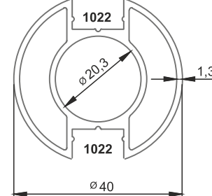
■ 2879 40'lık Çift Kanal Dikme Profili 1,3mm 0,755 kg/m
