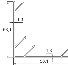
■ 7281 Kapak 0,580 kg/m
