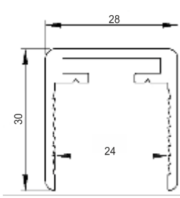
■ 7311 Cam U Profil 0,528 kg/m
