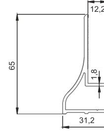
■ 4891 Alt Etek Profil Tekli 1,054 kg/m
