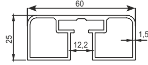
■ 4893 25x60 Kare Camlı Profil 12mm 0,931 kg/m
