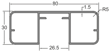
■ 12157 30x80 Kare Camlı Profil 26,5mm 1,076 kg/m
