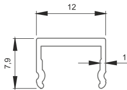
■ 592 Kare Dikme Kapak 0,073 kg/m
