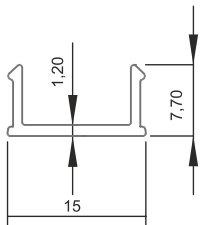
■ 7241 30x50 Dikme Kapağı 0,084 kg/m
