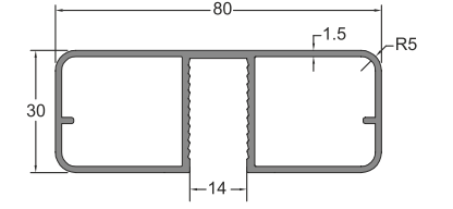
■ 12156 30x80 Kare Camlı Profil 14mm 1,092 kg/m
