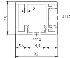
■ 4105 25x32 Kare Cam Profil 0,588 kg/m
