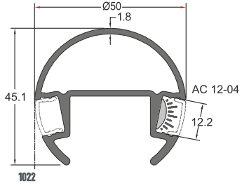
■ 12418 50'lık Ledli Boru 0,960kg/m
