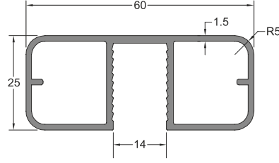
■ 12154 25x60 Kare Camlı Profil 14mm 0,829 kg/m
