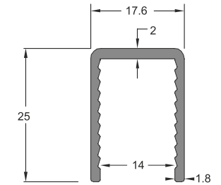
■ 12158 Cam Üst Profili 14mm 0,293 kg/m
