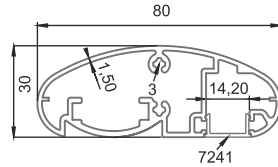
■ 7802 30x80 Elips Profil 1,221 kg/m
