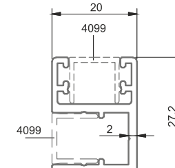
■ 4097 27x20 Kare Cam Profil 0,420 kg/m
