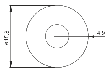
■ 916 16'lık Boru 4,9mm 0,454 kg/m
