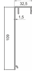
■ 3623 Zemin Üstü Cam Kanal Kapağı 0,683 kg/m
