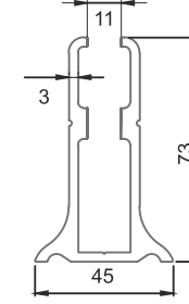
■ 822 Alt Etekli Profili 1,862 kg/m
