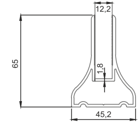
■ 4892 Alt Etek Profil Çiftli 1,196 kg/m
