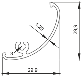
■ 7806 30x30 Elips Profil Kapağı 0,243 kg/m
