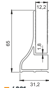
■ 4891 Alt Etek Profili Tekli 1,054 kg/m
