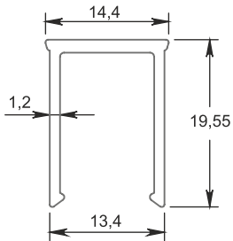
■ 7279 Kapak 0,175 kg/m
