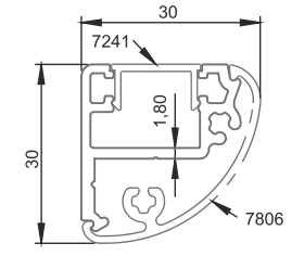
■ 7805 30x30 Elips Profil 0,405 kg/m
