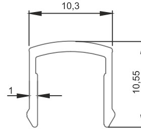
■ 1574 30'lık Kanallı Boru Kapağı 0,081 kg/m
