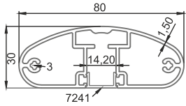
■ 7800 30x80 Elips Profil 1,221 kg/m
