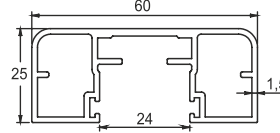
■ 6610 25x60 Kare Camlı Profil 24mm 0,887 kg/m
