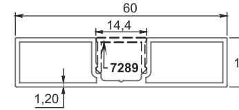
■ 7277 60x14 Çit Profili 0,523 kg/m
