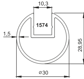
■ 1570 30'lık Kanallı Profil 1,5mm 0,467 kg/m
