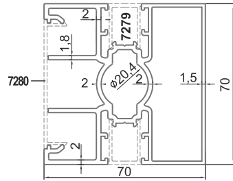
■ 12867 70x70 Çit Dikme Profili 2,303 kg/m
