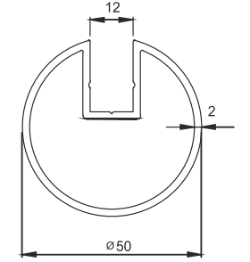
■ 4723 50'lık Kanallı Profil 2mm 1,026 kg/m
