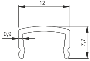
■ 1022 40'lık Dikme Kapağı 0,073 kg/m
