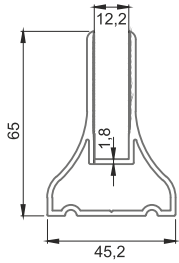
■ 4892 Alt Etek Profili Çift 1,196 kg/m
