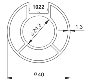
■ 2246 40'lık Tek Kanal Dikme Profili 1,3mm 0,806 kg/m
