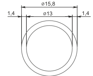
■ 2878 16'lık Boru 1,4mm 0,172 kg/m
