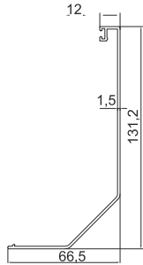
■ 10569 Yandan Montaj Cam Kanal Kapağı 0,809 kg/m
