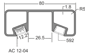
■ 12417 30x80 Kare Ledli Profil 26,5mm 1,289kg/m
