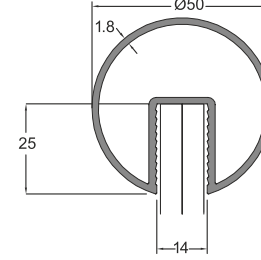
■ 12152 50'lık Kanallı 14mm 1,003kg/m
