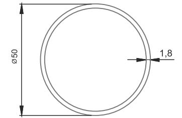
■ 2984 50'lık Boru 1,8mm 0,738 kg/m
