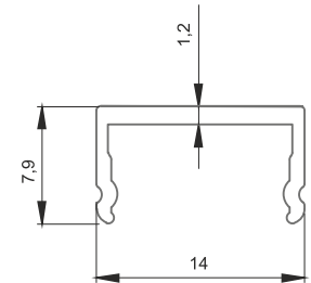
■ 1411 Kare Dikme Kapak 0,080 kg/m
