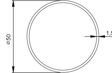
■ 2622 50'lık Boru 1,5mm 0,620 kg/m
