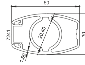
■ 7804 30x50 Elips Tek Kanal Dikme Profili 0,900 kg/m
