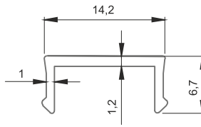
■ 4112 Kapak 0,078 kg/m
