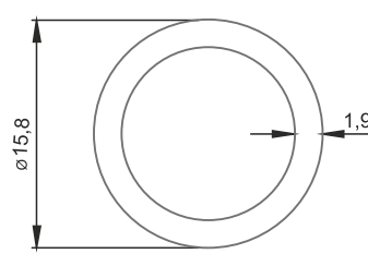
■ 1234 16'lık Boru 1,9mm 0,224 kg/m
