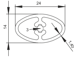
■ 7808 14x24 Elips Profil 0,289 kg/m
