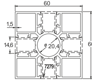
■ 7271 60x60 Çit Dikme Profili 1,937 kg/m
