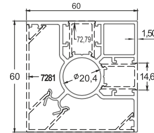
■ 7272 60x60 Çit Dikme Profili 1,376 kg/m
