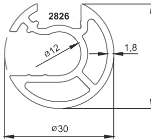
■ 2825 30'lık Dikme Profili Camlı 1,8mm 0,598 kg/m
