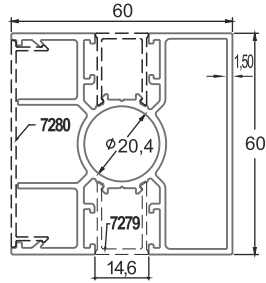
■ 7270 60x60 Çit Dikme Profili 1,639 kg/m
