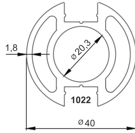
■ 1010 40'lık Çift Kanal Dikme Profili 1,8mm 1,143 kg/m
