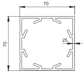
■ 4117 70x70 Profil 2,439 kg/m
