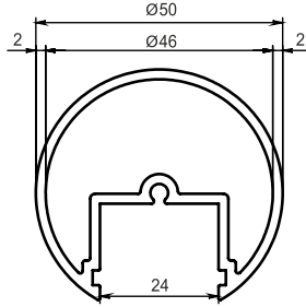
■ 3809 50'lik Kanallı Boru 24mm 1,050 kg/m
