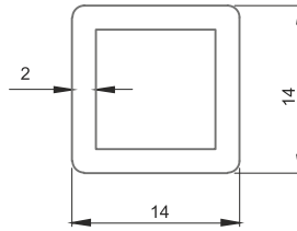
■ 1409 14x14 Kare Profil 0,258 kg/m
