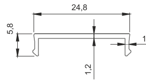
■ 4113 Kapak 0,108 kg/m
