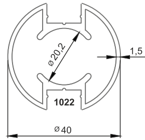
■ 1599 40'lık Çift Kanal Dikme Profili 1,5mm 0,762 kg/m
