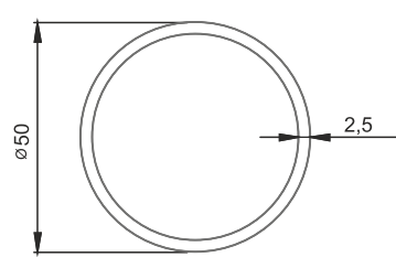
■ 917 50'lık Boru 2,5mm 1,011 kg/m
