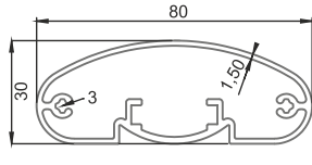
■ 7801 30x80 Elips Profil 1,099 kg/m
