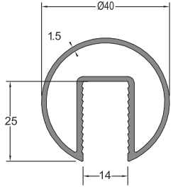
■ 12150 40'lık Kanallı 14mm 0,729 kg/m
