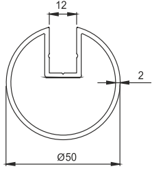
■ 4723 50'lik Kanallı 12mm 1,026 kg/m
