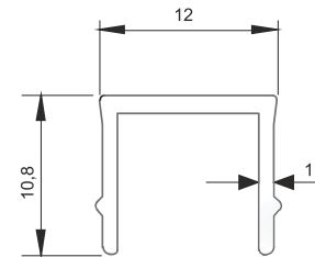
■ 4099 Kapak 0,094 kg/m
