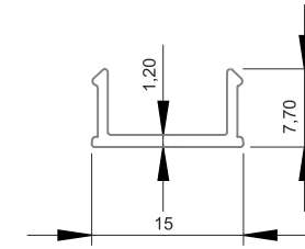
■ 7241 Kapak 0,084 kg/m
