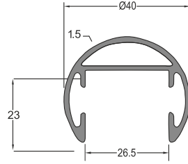
■ 12151 40'lık Kanallı 26,5mm 0,621 kg/m
