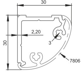
■ 7807 30x30 Elips Profil 0,389 kg/m
