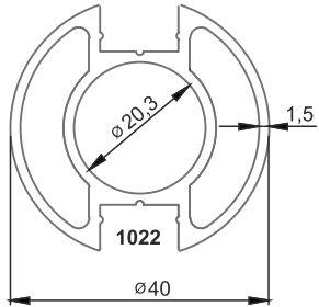
■ 1565 40'lık Çift Kanal Dikme Profili 1,5mm 0,911 kg/m
