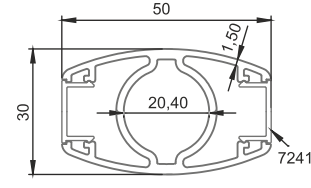
■ 7803 30x50 Elips Çift Kanal Dikme Profili 0,864 kg/m
