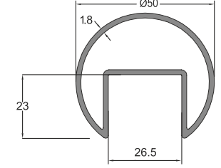
■ 12153 50'lık Kanallı Boru 26,5mm 0,946kg/m
