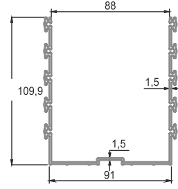
■ 6603 Zemin Altı Kanal Profili 1,806 kg/m
