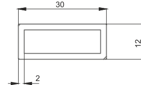
■ 10059 12x30 Kare Profil 0,411 kg/m
