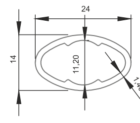
■ 7809 14x24 Elips Profil 0,230 kg/m
