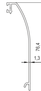
■ 11494 Zemin Üstü Cam Kanal Profili 0,370 kg/m
