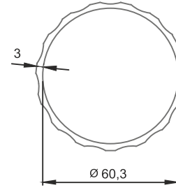
■ 1036 65'lık Tırtıllı Boru 1,377 kg/m
