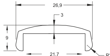
■ 12281 Cam Üst Profili 0,234kg/m
