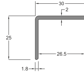
■ 12159 Cam Üst Profili 26,5mm 0,382 kg/m
