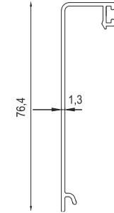
■ 11495 Zemin Üstü Cam Kanal Profili 0,395 kg/m
