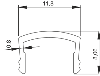
■ 2826 30'lık Dikme Kapağı 0,072 kg/m
