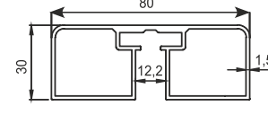
■ 4894 30x80 Kare Camlı Profil 12mm 1,187 kg/m
