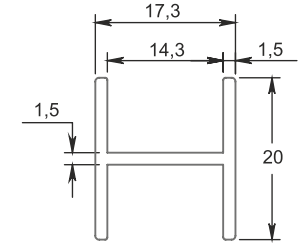
■ 7278 20x17,3 Çit Profili 0,220 kg/m
