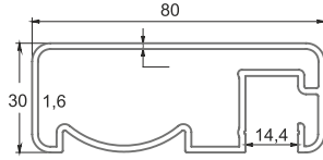
■ 1000 30x80 Kare Profil 1,149 kg/m
