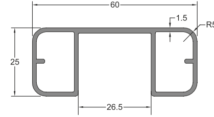
■ 12155 25x60 Kare Camlı Profil 26,5mm 0,781 kg/m
